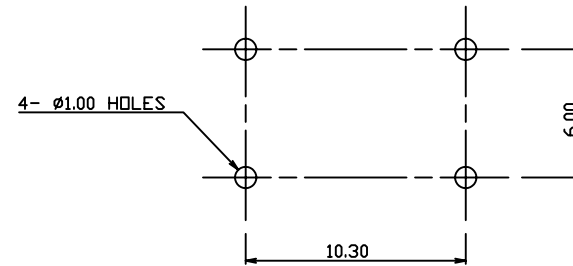
P.C.B DIMENSION
