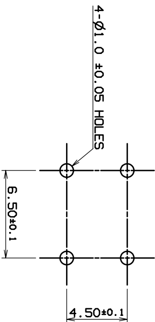
P.C.B DIMENSION
