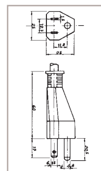
P620 UL 817
