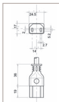
PA85 EN 60320 -1
