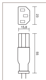
PA99 UL 817
