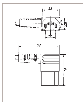
PW80 EN60320 -1
