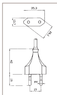
E 73 CEE7/XVII
