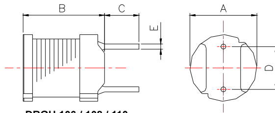
DRGH 106 / 108 / 110
