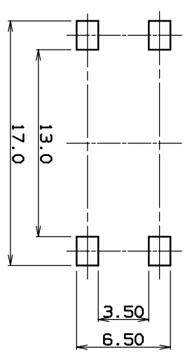
P.C.B DIMENSION
