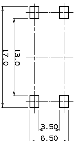
P.C.B DIMENSION
