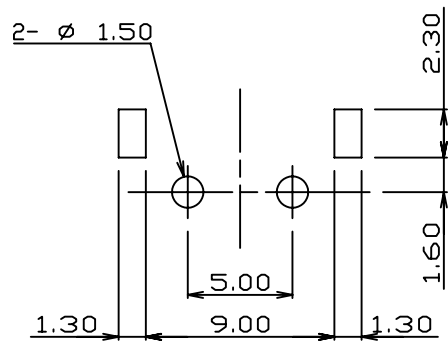
P.C.B DIMENSION
