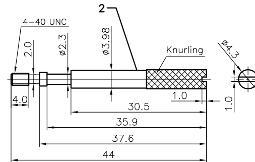
Long BOLT
