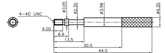
Long BOLT
