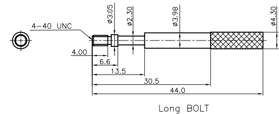
Long BOLT
