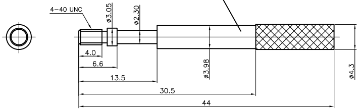
Long BOLT
